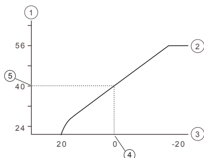
Rys. 6: Ustawiona wartość 40 dla parametru KRZYWA
